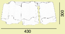
MX6357-60-3 Plafon de tres pantallas A -19 3 x 60W Material: Hierro y Vidrio Dimensión de caja: 89.0X30.0X39.0cm Contenido: 1 pieza / caja
