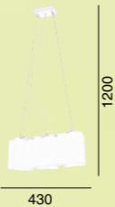
MD998-3 Colgante de tres pantallas A -19 3 x 60W Material: Hierro y Vidrio opalino Dimensión de caja: 77.0X26.0X32.0cm Contenido: 1 pieza / caja
