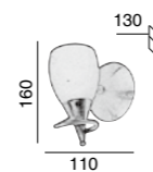
549 ST/OPF 127V E12 1x40W
